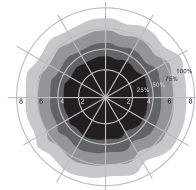
Detectiebereik plafondmontage (Eenheid: m) Voorgestelde montagehoogte: 2,5 - 6m
